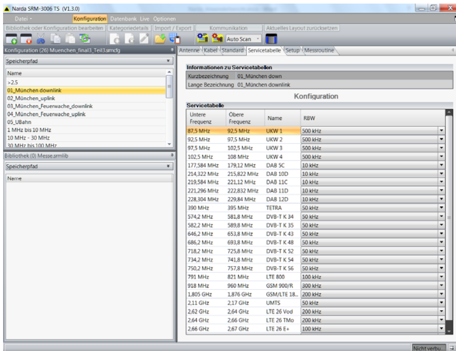
Figure 3: Beispielhaft – Servicetabelle für Sendeanlagen nach der derzeitigen Frequenzbelegung in Deutschland – für die Region München konkretisiert
