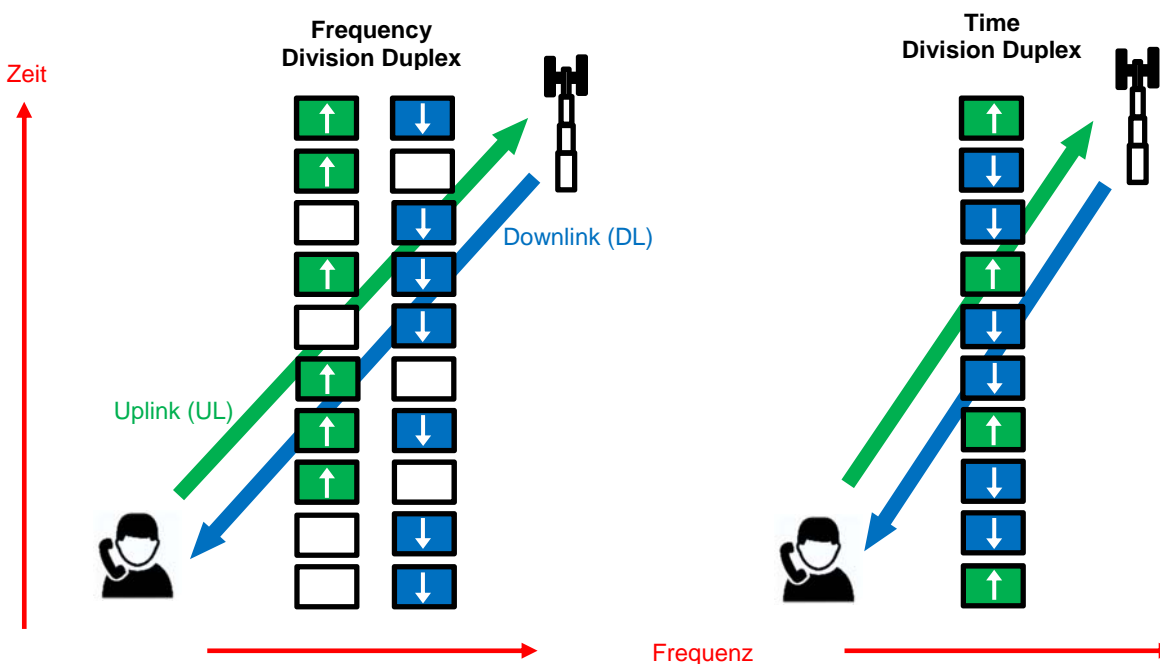
Bild 2: Unterscheidung FDD (links) und TDD (rechts)
