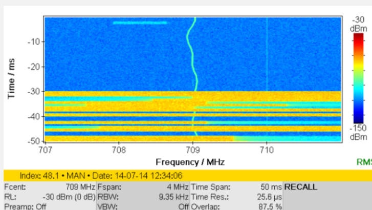
Abb. 5: Zeitlich lückenloses HighRes-Spektrogramm entlarvt die Emissionen eines Folienschweißgerätes zwischen LTE-Nutzsignalen
