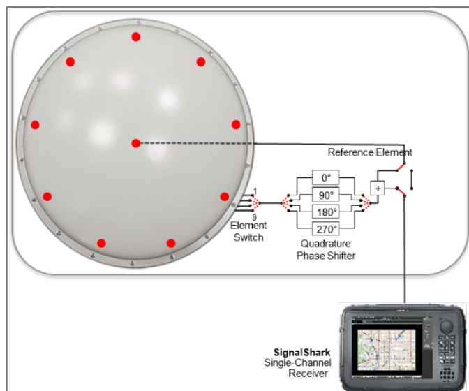
Abb. 2. Prinzipieller Aufbau der einkanaligen Peilantenne ADFA.
