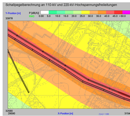
Abb. 7. Schallpegelberechnung 1 m über dem Boden
