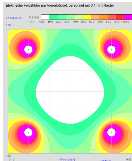
Abb. 6. Randfeldstärken am Viererbündel
