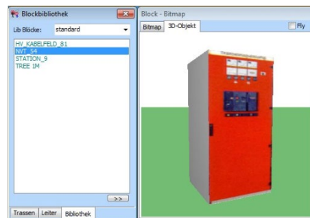
Abb. 1. Bauteilbibliothek
