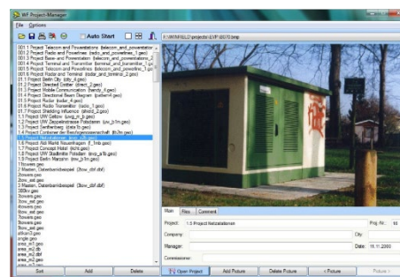
Abb. 3. Projektarchivierung
