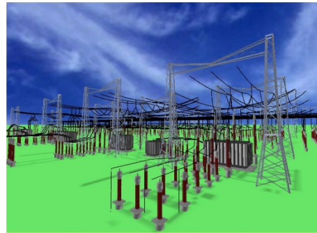
Abb. 4. Magnetisches Feld an einer Schaltanlage
