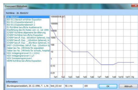
Abb. 2. Integrierte Grenzwertbewertung
