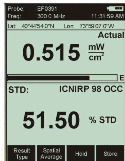
标准采用：当使用计权探头测量时，通过简单地设置频率并选择 NBM-550 内置的标准（如 ICNIRP 标准），就可得到计权测量结果。如果场强来源主要是已知的某个单一频率，这种评估非常有用。即使使用普通探头进行测量，也可以显示相对于标准限值的百分比结果。所有标准参见第 6 页。
