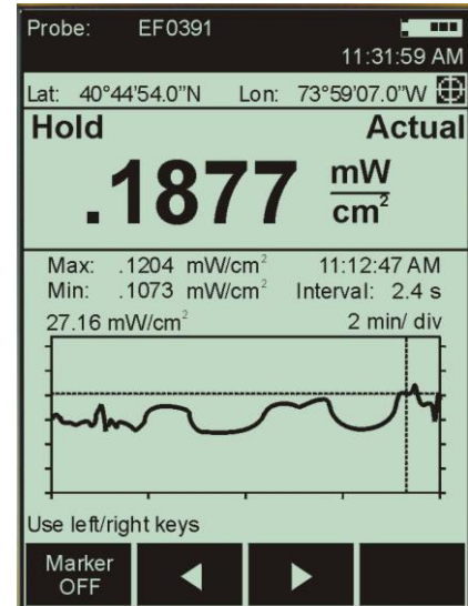
历史记忆模式显示场强随时间变化的曲线，可用标识线读取显示特定时刻的场强值
