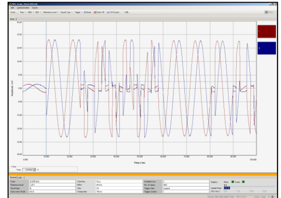
Scope-Ansicht für eine detaillierte Analyse über der Zeit (Bildschirm der NRA Scope Demo Software)
